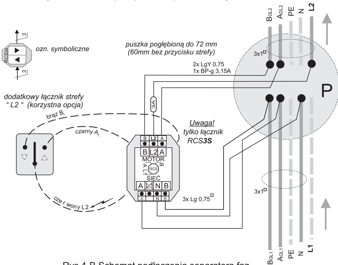
Rys.4-B Schemat podłączenia separatora faz - opcjonalnie jako separatora strefy sterowania
