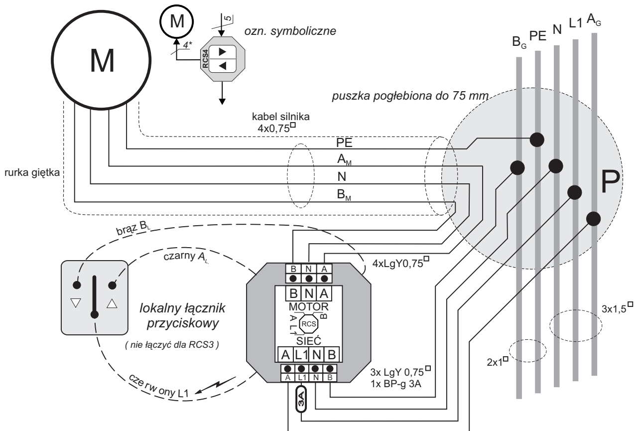
Rys.2-B Schemat podłączenia pojedynczego napędu
