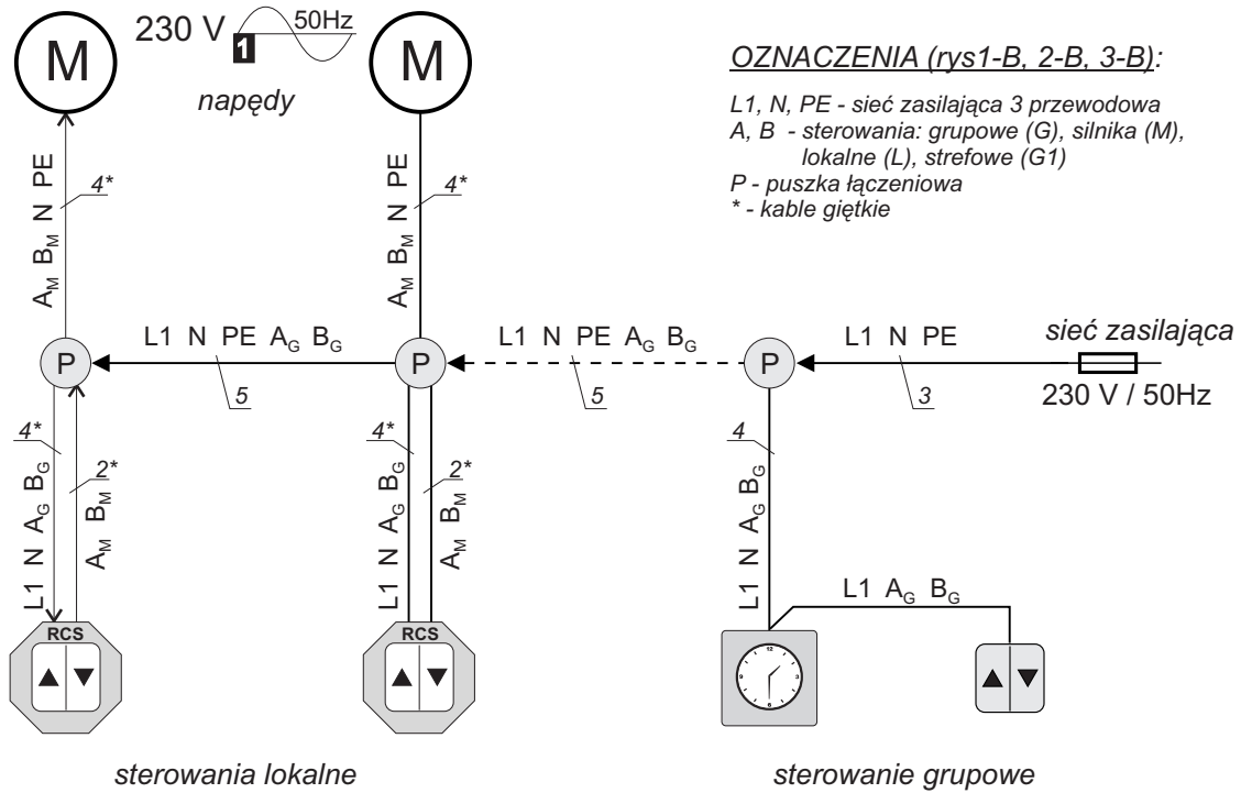
Rys.1-B Poglądowy schemat instalacji z RCS4,5
