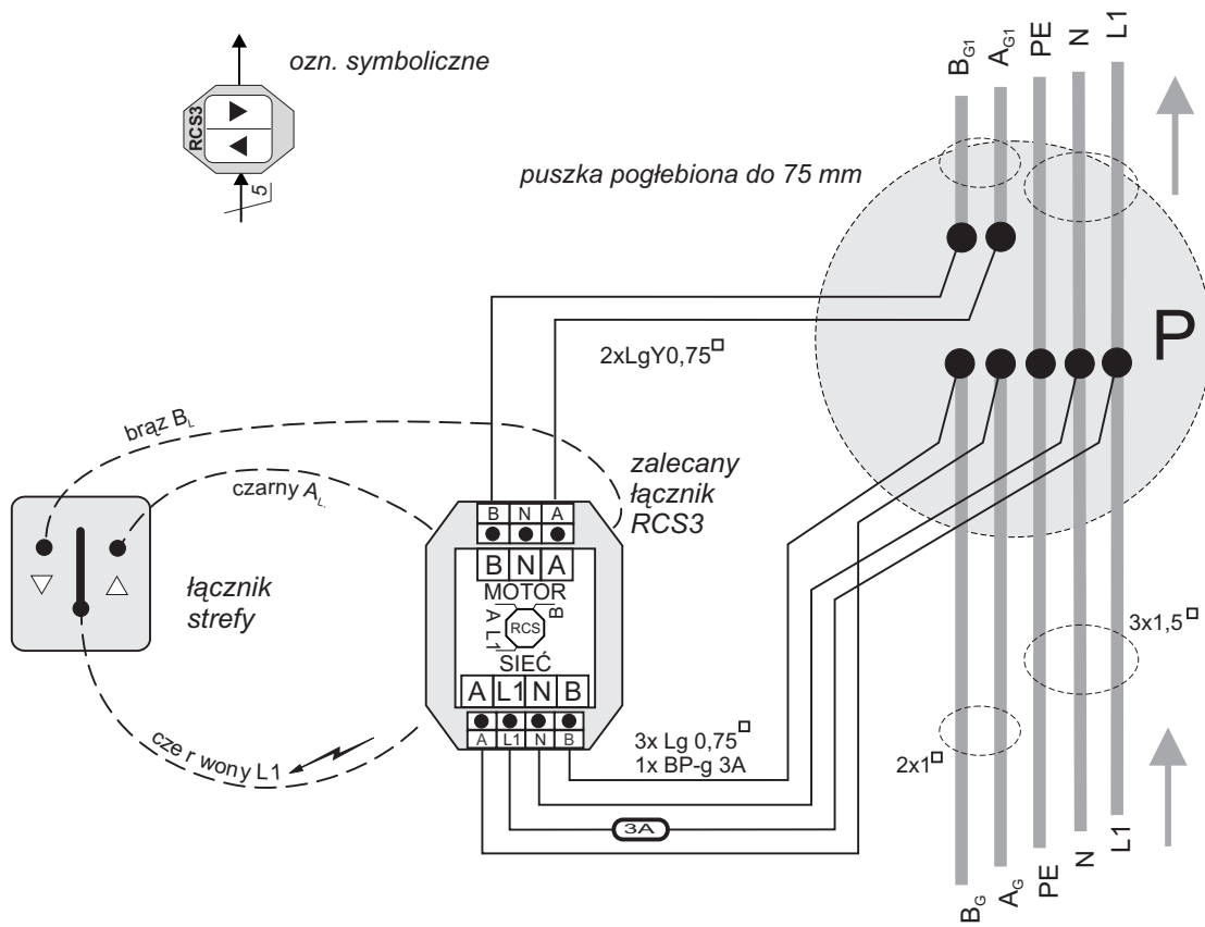
Rys.3-B Schemat podłączenia separatora strefy
