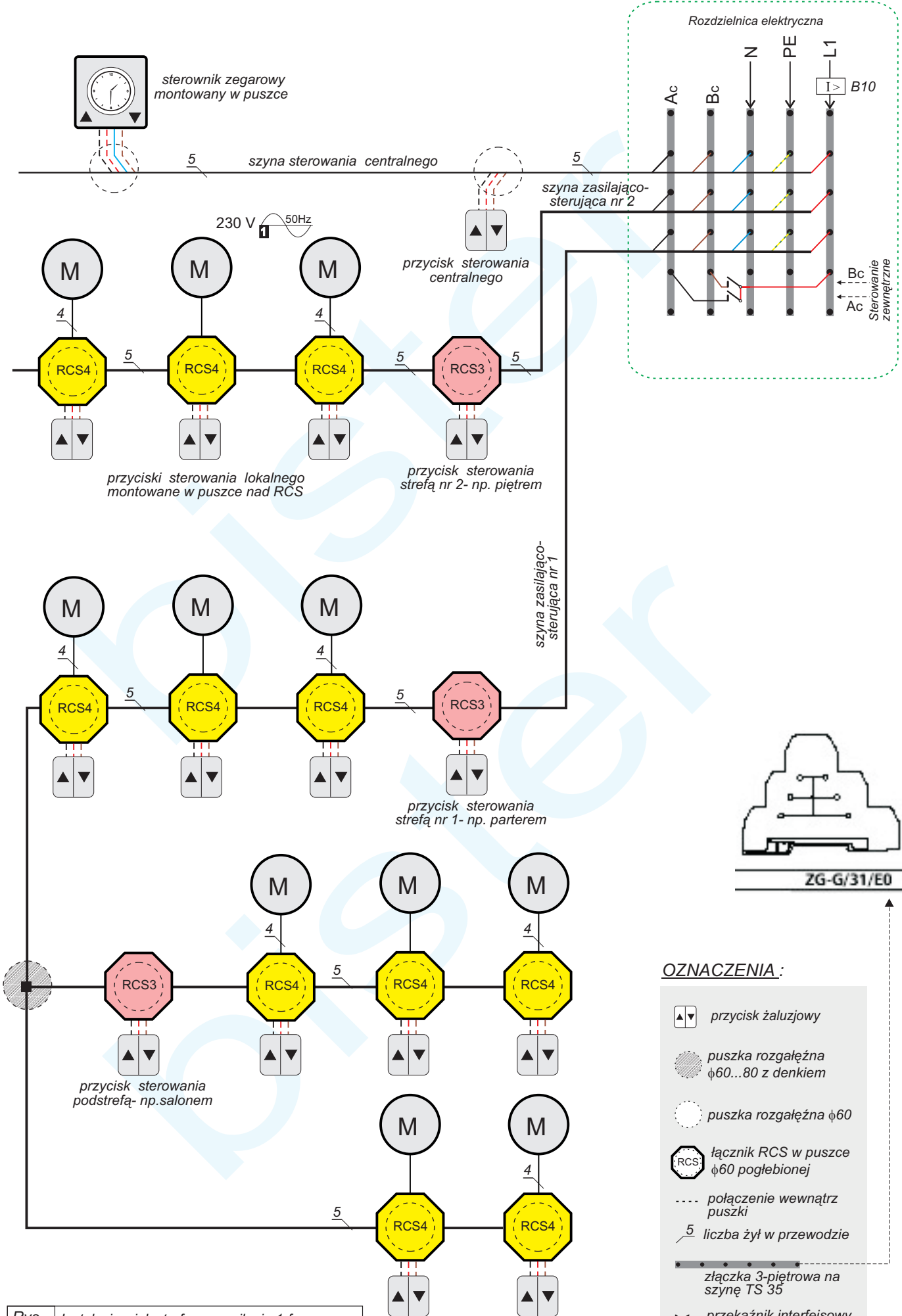
Rys. 0902 Instalacja wielostrefowa, zasilanie 1-fazowe. Strefowanie na szynach zasilająco-sterujących.
