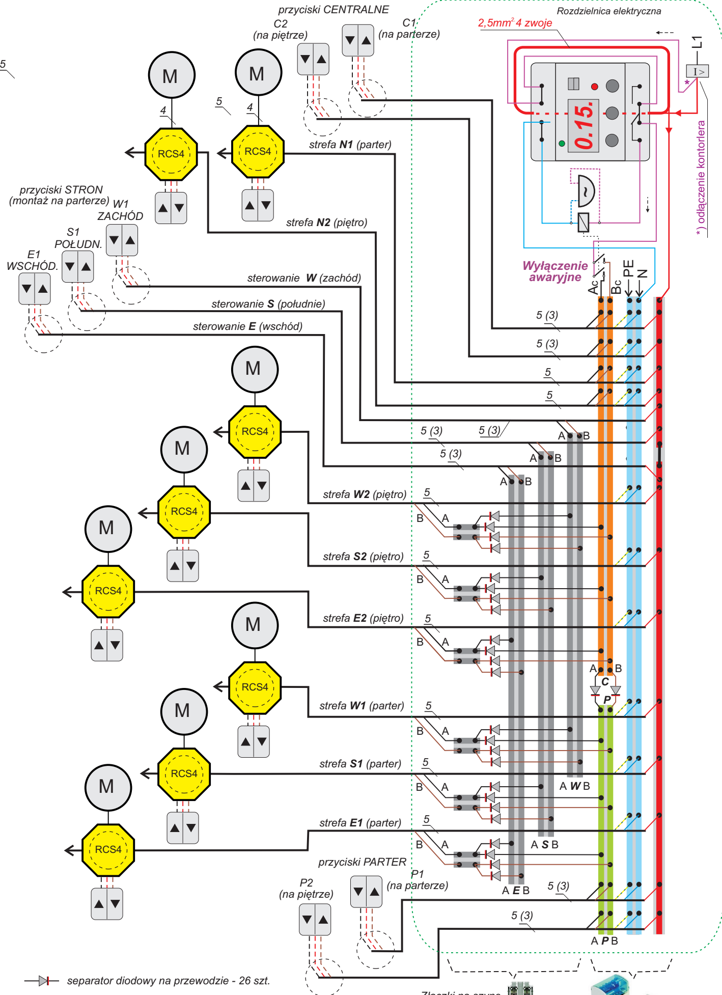
Rys. 1701 Instalacja wielostrefowa z kontrolerem OM-110, zasilanie 1-fazowe. Budynek: parter (1)+ piętro (2). Sterowanie: centrale (C), strefa parter (P), 3 strefy stron światła (W, S, E). Strona N - tylko centralne.
