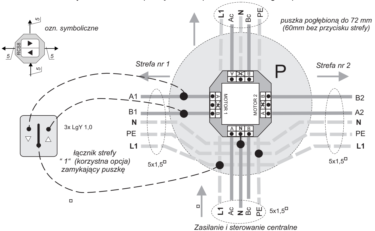
Rys.7-B Schemat podłączenia łącznika RCS8 jako separatora dwóch stref
