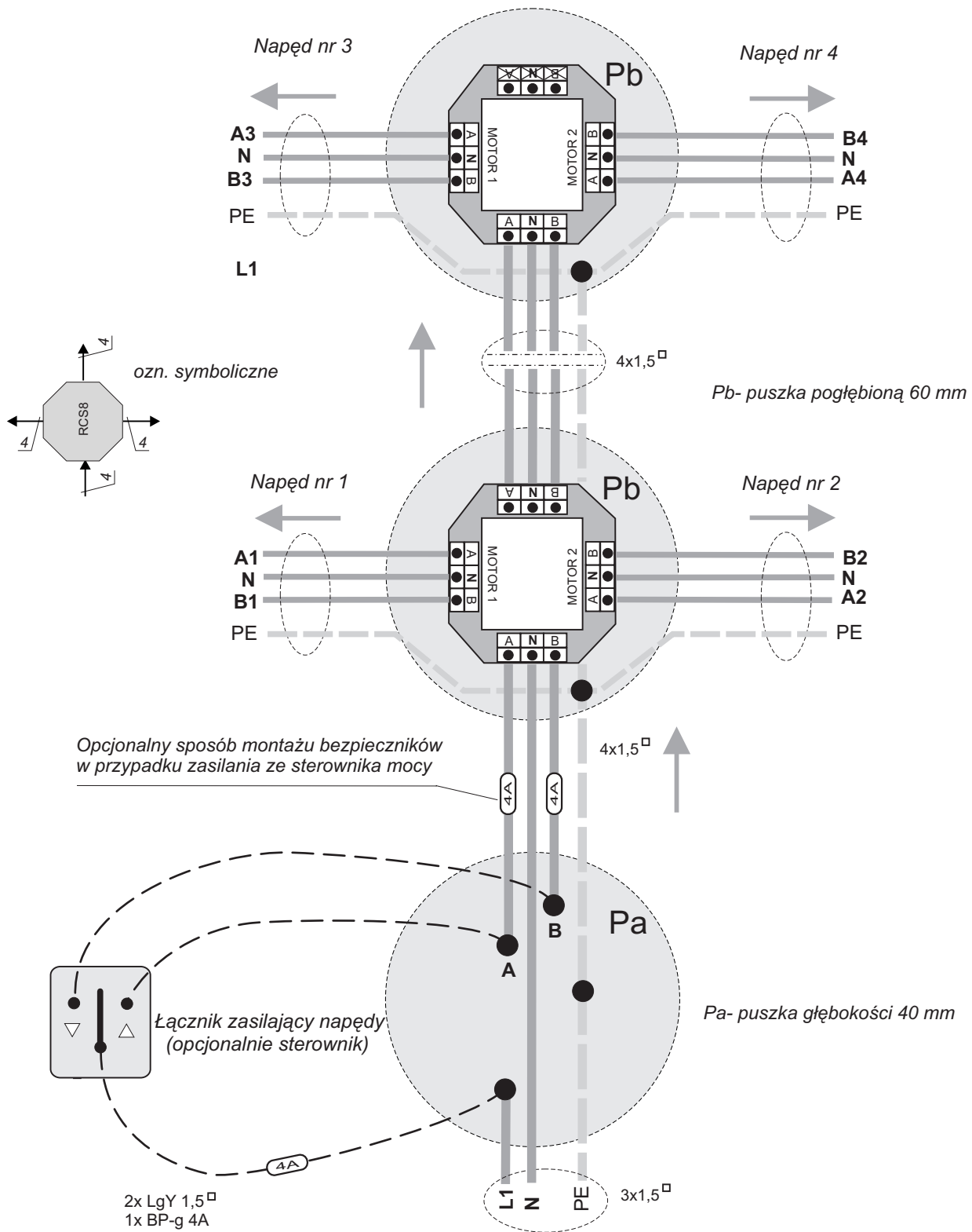
Rys.8-B Schemat podłączenia łącznika RCS8 jako separatora 2 (4) napędów z mechanicznym wyłącznikiem krańcowym
