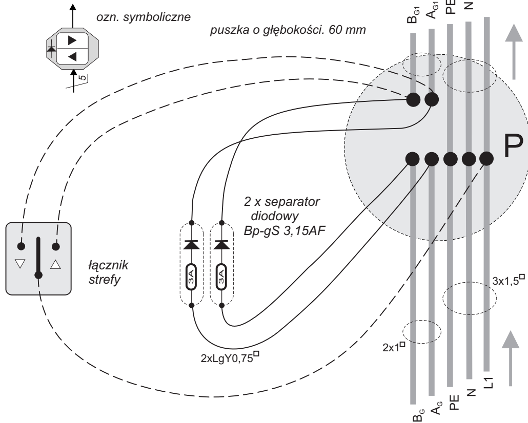
Rys.6-B Schemat podłączenia separatora diodowego w puszce
