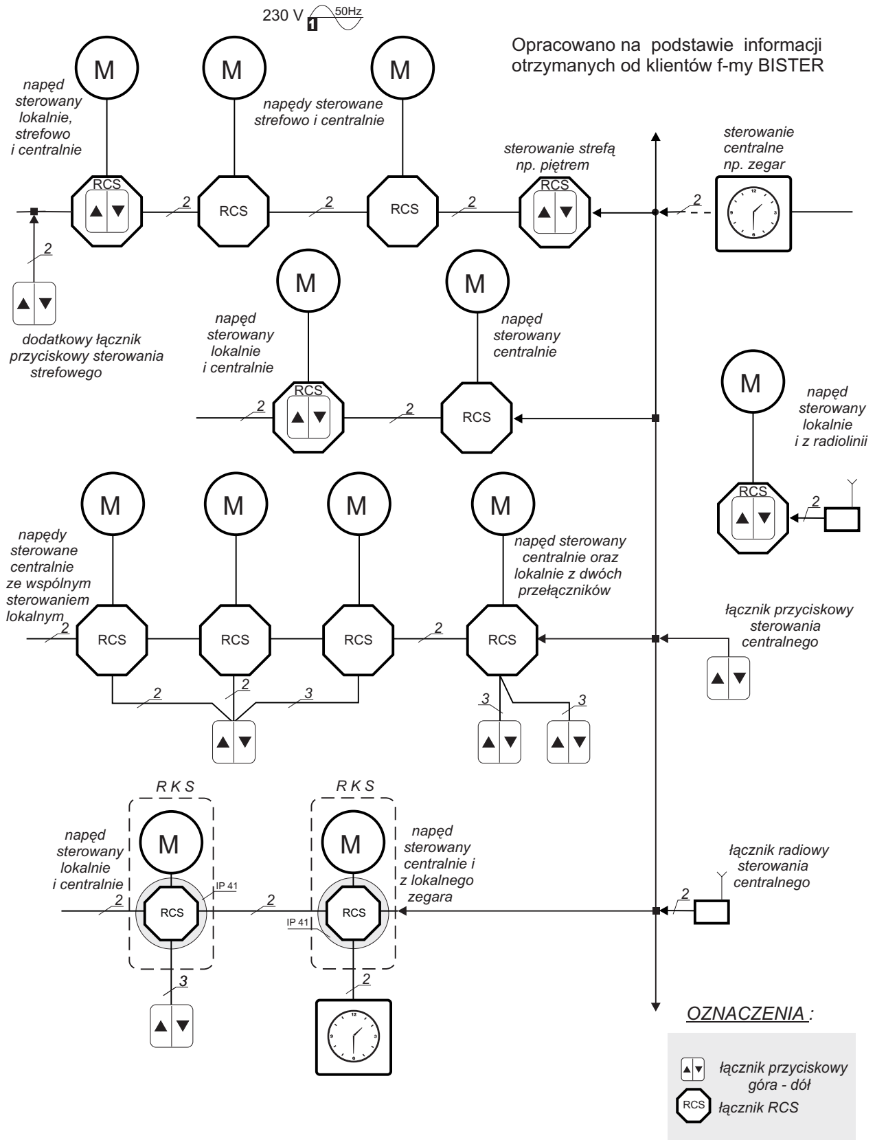
Rys.5-B Przykładowe konfiguracje połączeń instalacji napędu rolet (nie uwidoczniono linii zasilania L1, N, PE)
