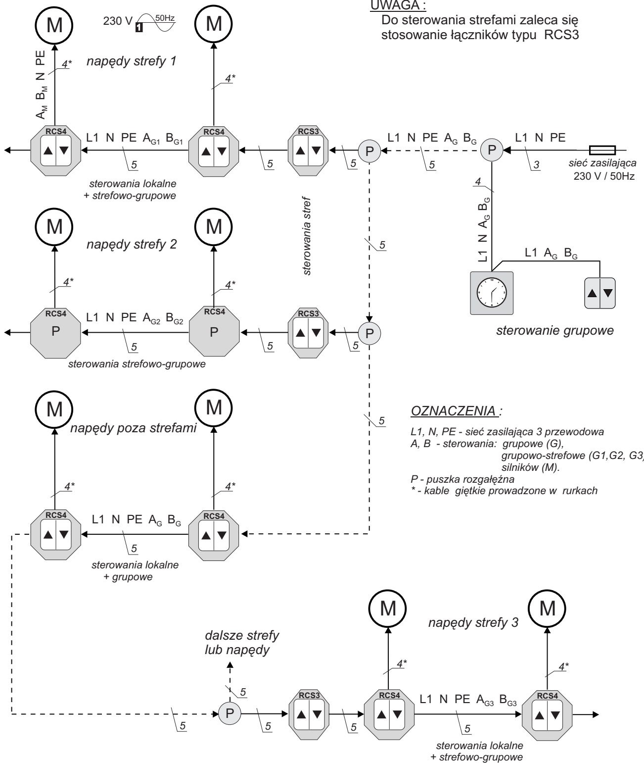
Rys.4-B Poglądowy schemat przykładowej instalacji strefowanej
